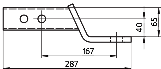
00045503 Кронштейн 50x50 для фаркопа универсальный
